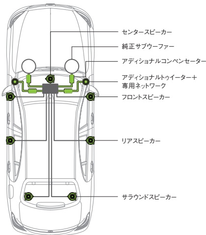
SC-213Mb 9スピーカーモジュール システム構成図
