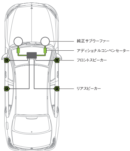
SC-222M4 4スピーカーモジュール システム構成図
